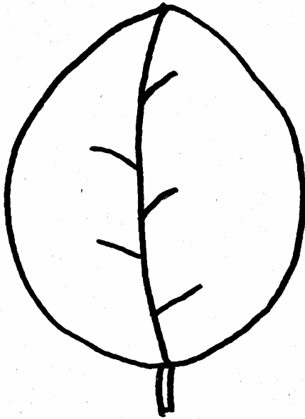
1 breit eiförmig
