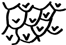
5 mittel
