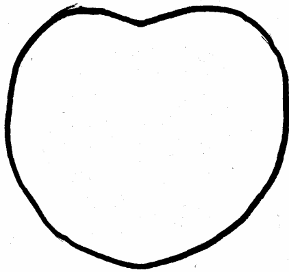
1 kreisförmig
