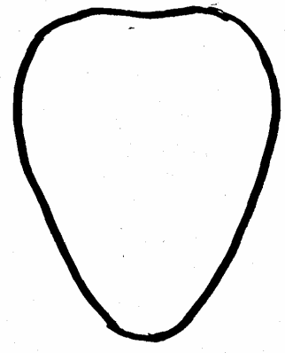
3 kegelförmig
