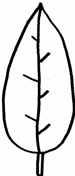
3 schmal eiförmig
