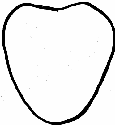
4 breit kegelförmig
